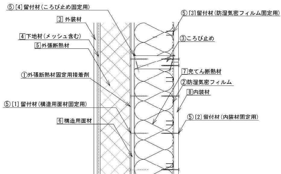
鉛直断面詳細図
